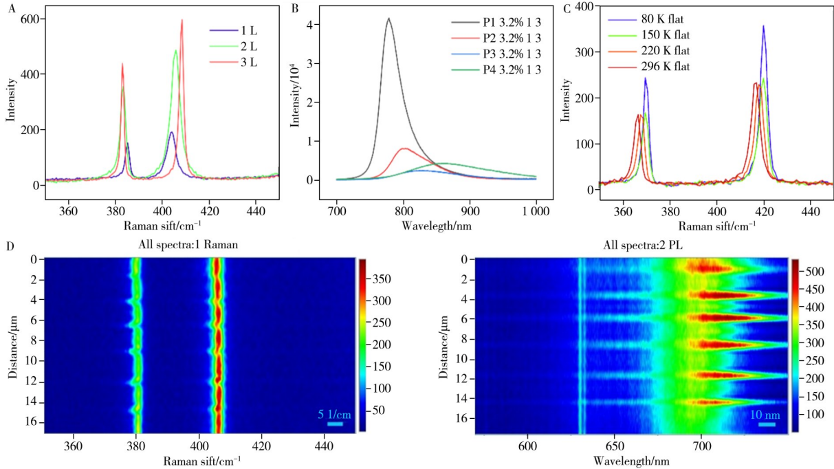
图2 MoS 2 的拉曼、PL光谱与扫描结果图
